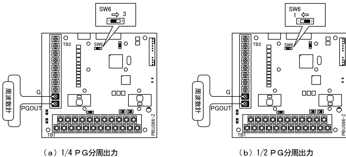
図6. 4 PG出力
