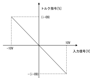
図 5. 5 アナログ入カートルク指令特性
