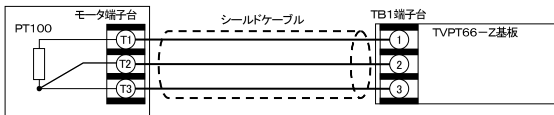
図4. 1 TVPT66-ZとPT100測温体との接続（3芯ケーブルの場合）
