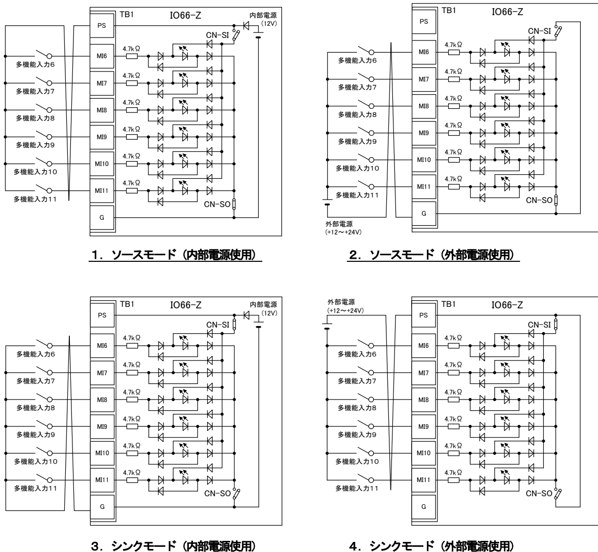
図4. 1 多機能入力の接続
