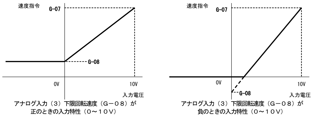
図5. 8 電圧入力0～10Vの速度指令特性
