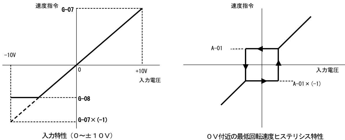
図5. 7 電圧入力0～±10Vの速度指令特性
