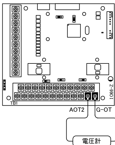
図 5. 9 アナログ出力（２）の接続例
