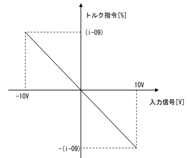
図5.5 アナログ入力トルク指令特性
