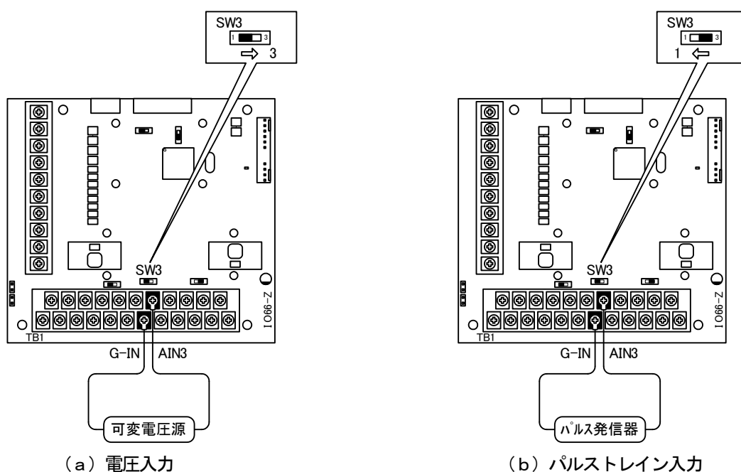
図 5. 6 アナログ入力 (3) の接続例
