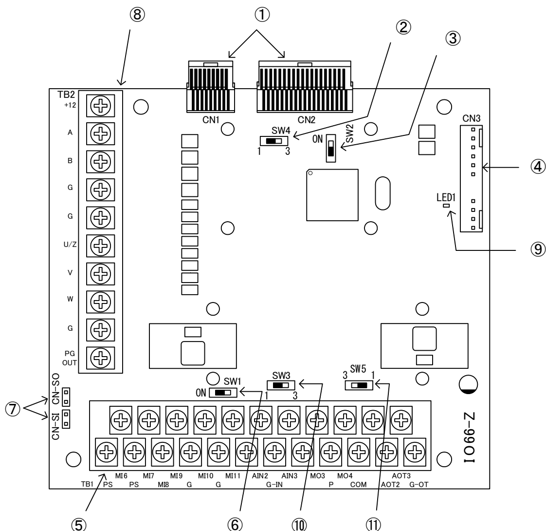
図3. 1 IO66-Z基板
