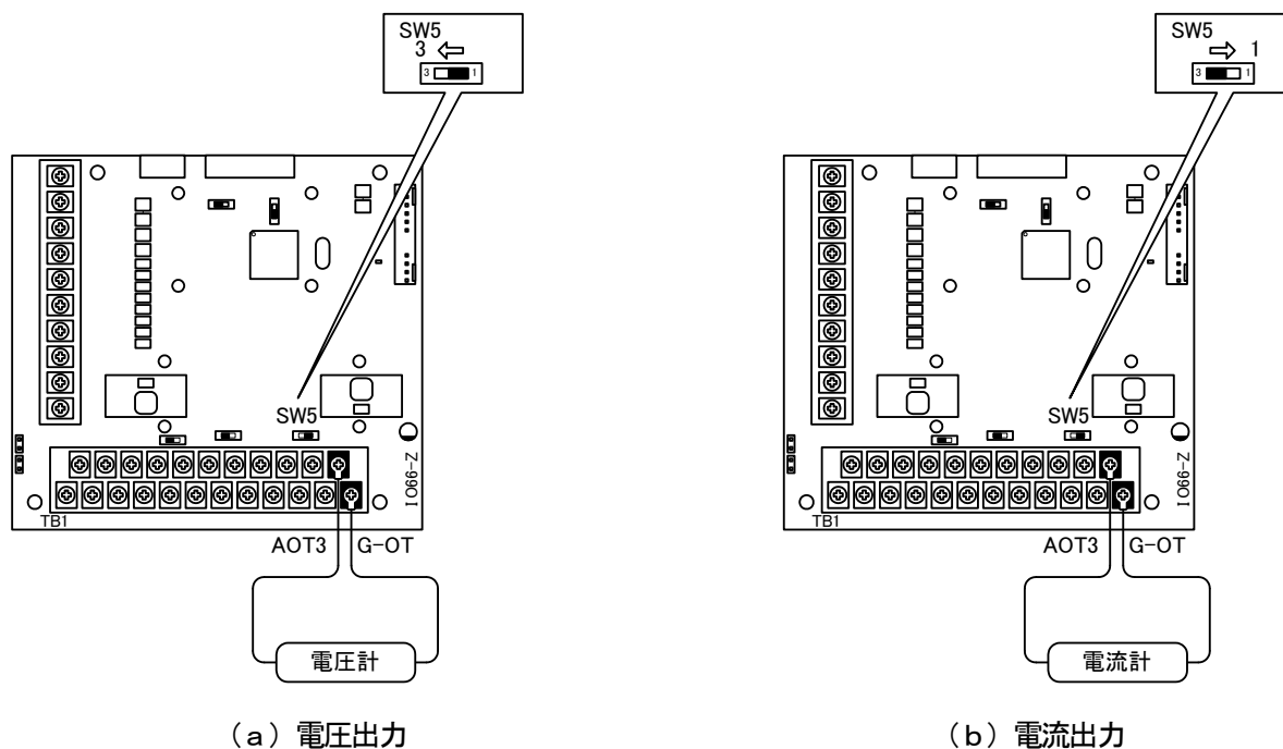
図 5. 10 アナログ出力（3）の接続例
